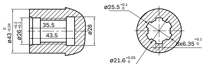
SHAFT E
