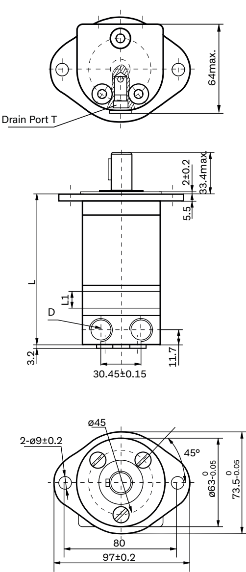
Flange F
