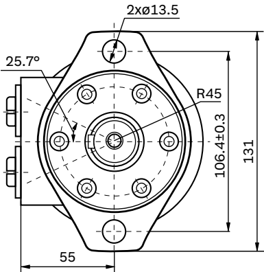
Flange 2
