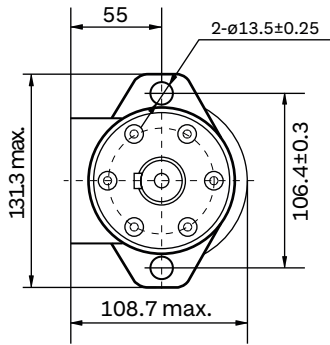
Flange 2
